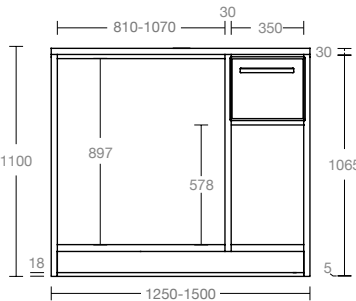
BASE PER MACCHINA CAFFÈ COFFEE MACHINE UNIT
