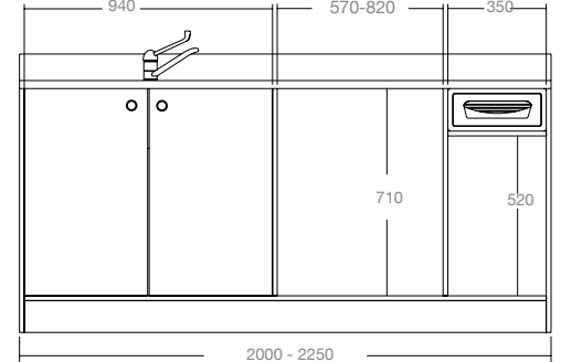
MODULO MACCHINA CAFFÈ RETRO COMBI CON 2 LAVELLI CAFFÈ MACHINE BACKCOUNTER COMBI WITH 2 SINK
