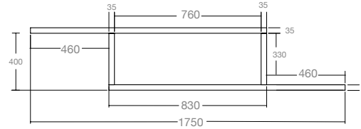
RETROALZATA BOTTIGLIERA ZETA P 236 ZETA BOTTLE COMPARTMENT D 236
