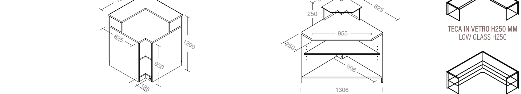
ANGOLO ESTERNO BAR 90° L1000 H1200 P1000 MM EXTERNAL BAR CORNER 90° W1000 H1200 D1000 MM ANGOLO INTERNO BAR 90° L925 H1200 P925 MM INTERNAL BAR CORNER 90° W925 H1200 D925 MM TECA IN VETRO H250 MM LOW GLASS H250 CASTELLO VETRI H400 MM FRAME GLASS H400
