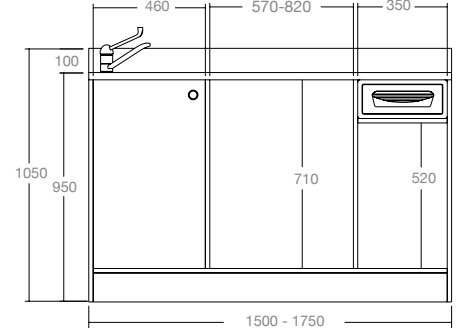
MODULO MACCHINA CAFFÈ RETRO COMBI CON 1 lavello CAFFÈ MACHINE BACKCOUNTER COMBI WITH 1 SINK
