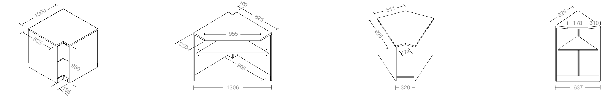
ANGOLO ESTERNO 90° L1000 H950 P1000 MM EXTERNAL CORNER 90° W1000 H950 D1000 MM ANGOLO INTERNO 90° L925 H950 P925 MM INTERNAL CORNER 90° W925 H950 D925 MM ANGOLO ESTERNO 45° L945 H950 P825 MM EXTERNAL CORNER 45° W945 H950 D825 MMMM ANGOLO INTERNO 45° L795 H950 P825 MM INTERNAL CORNER 45° W795 H950 D825 MM
